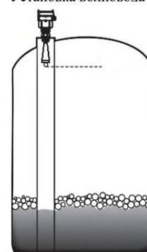
Установка волновода
